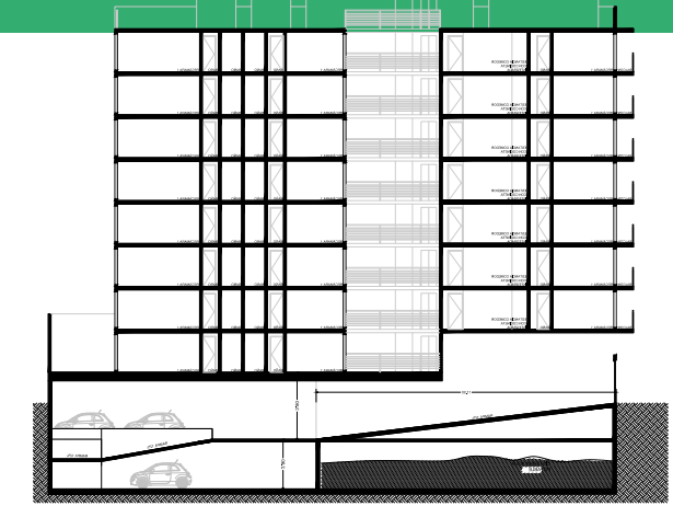
CORTE ESQUEMATICO
