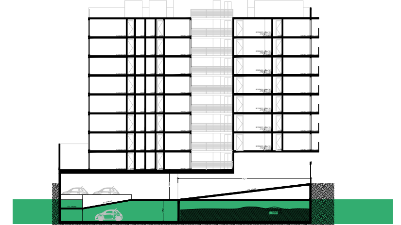
CORTE ESQUEMATICO
