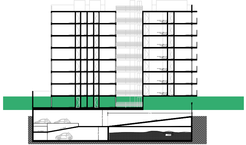
CORTE ESQUEMATICO
