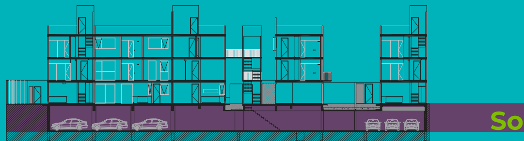
CORTE ESQUEMÁTICO
