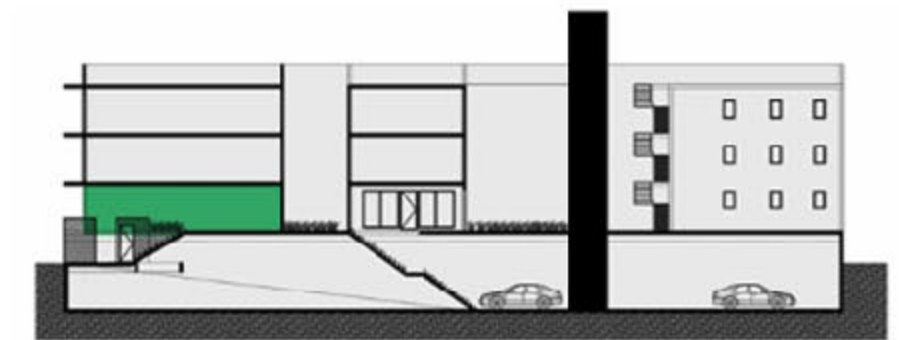
SECCIÓN ESQUETÁTICA
